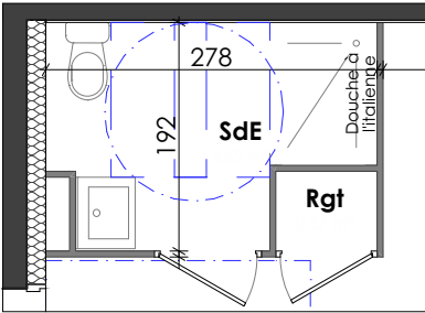
Plan réversibilité salle d'eau PMR
