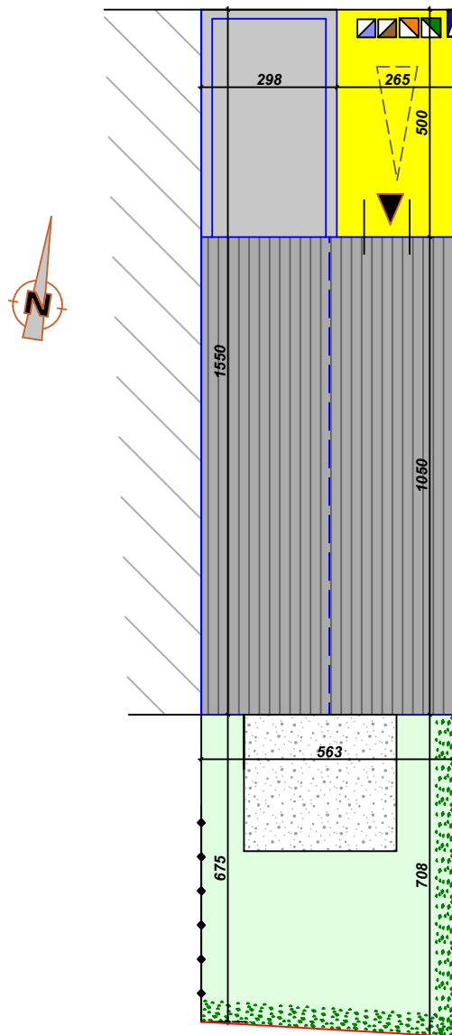
PLAN MASSE - Ech: 1/150
