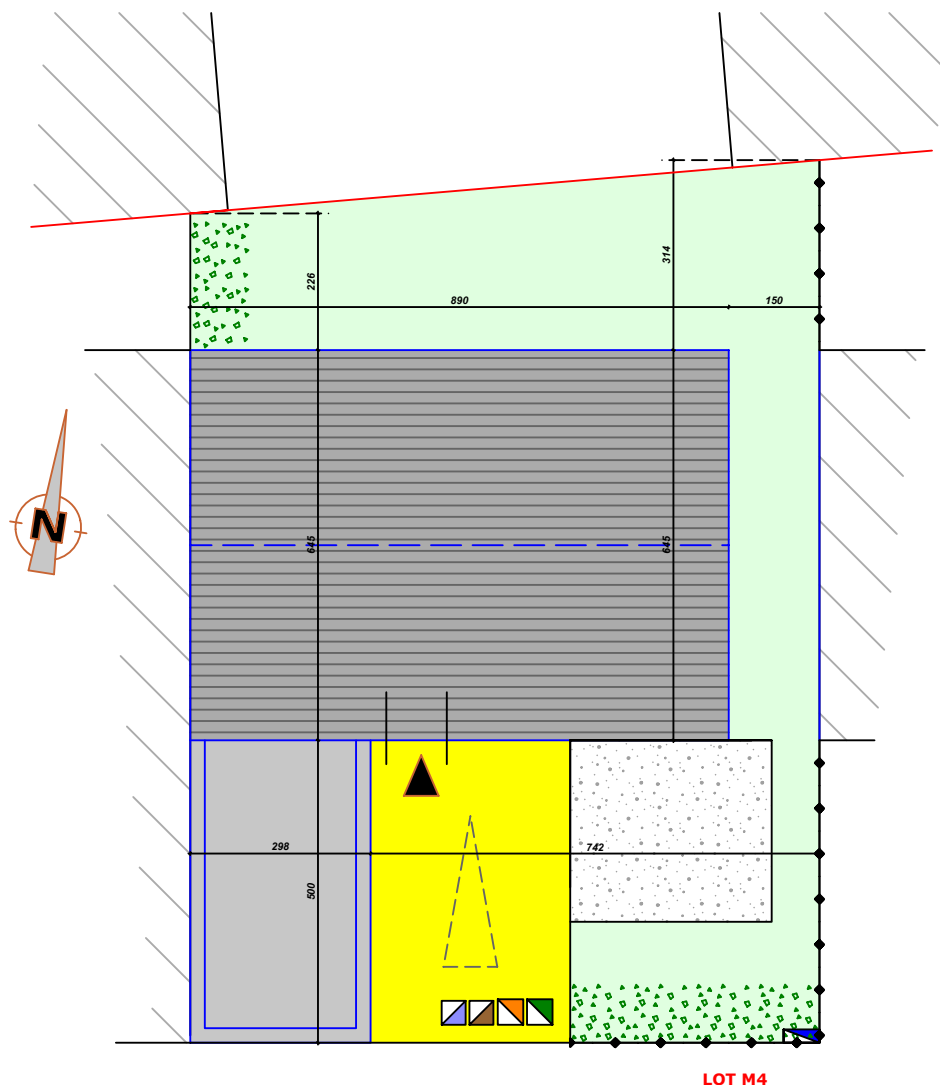
PLAN MASSE - Ech: 1/125
