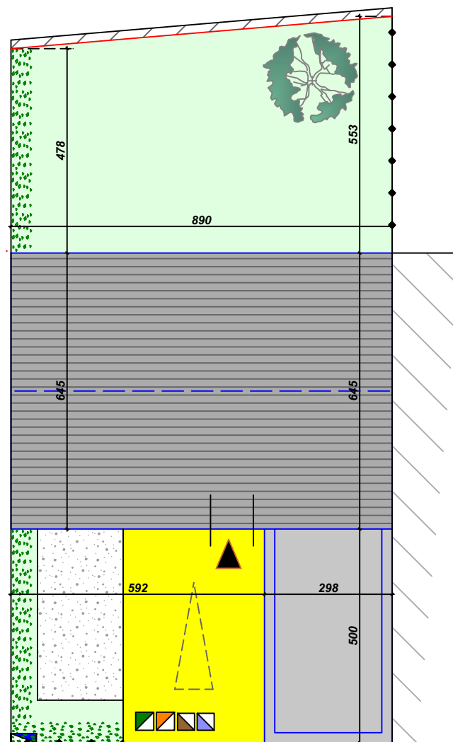
PLAN MASSE - Ech: 1/125
